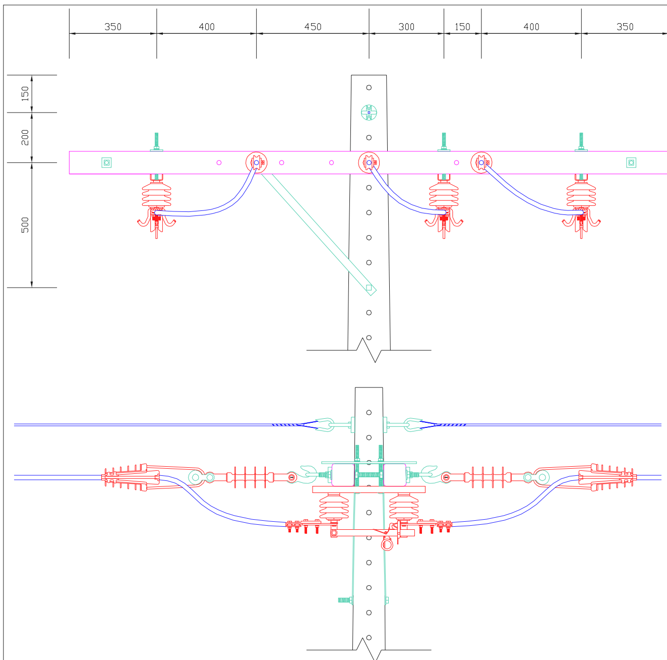
Instalação com chave faca para manobra
